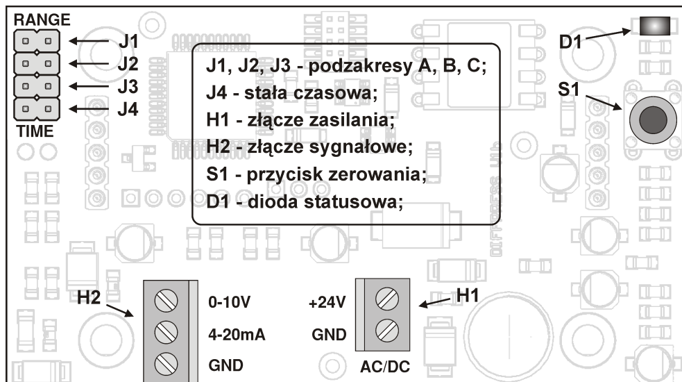
Rysunek 3. Opis wyprowadzeń przetwornika różnicy ciśnienia.
